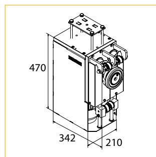
27. RTD 3000
