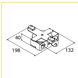
22. Return Pulley
