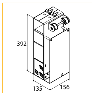
26. RTD 1000
