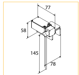
30. Limit Switch Set
