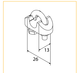
22. Rope Clamp
