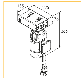
26. RTD 1100
