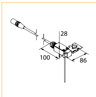
27. Limit Switch Set
